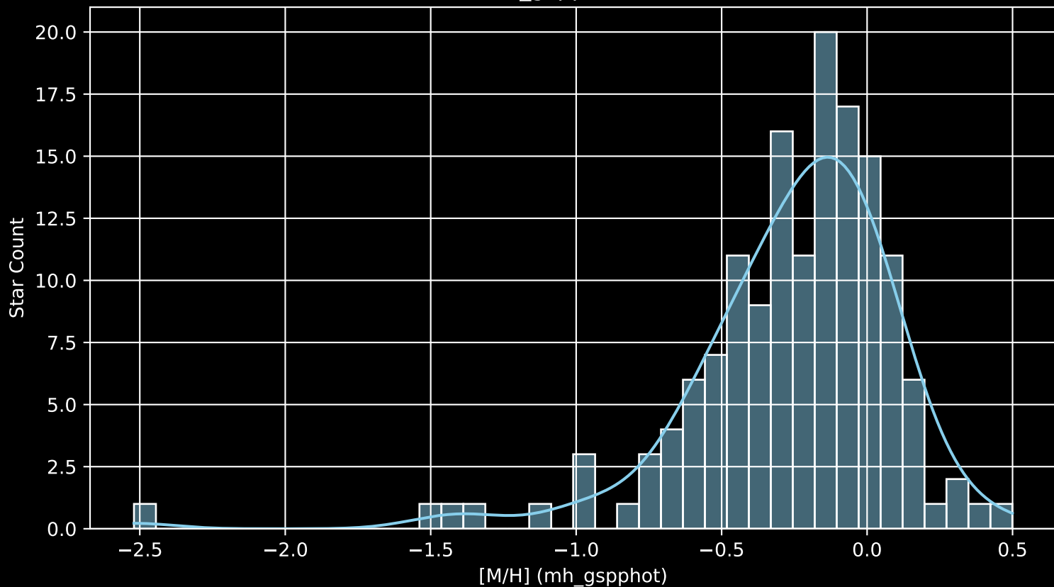
APOGEE DR17 Field: [040+43 MGA [M/H] (mh_gspphot) (n= 150)
